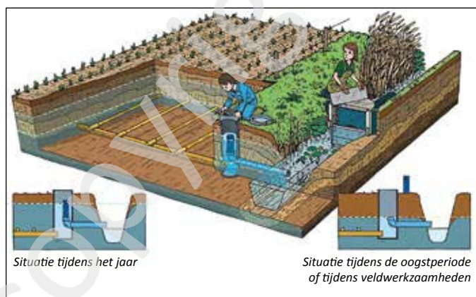
Figuur 1. - Illustratie van de werking van een peilgestuurde drainage (Bron: Boeren Natuur Vlaanderen)
