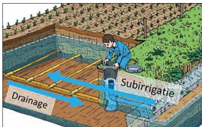
Figuur 2. - Het concept van drainage en subirrigatie. Bij peilgestuurde drainage stroomt het water van het perceel naar de gracht. Bij subirrigatie infiltreren het water van de gracht in het perceel. (Bron: Boeren Natuur Vlaanderen)
